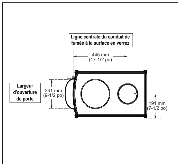
Figure 3.3 – Vue de dessus
