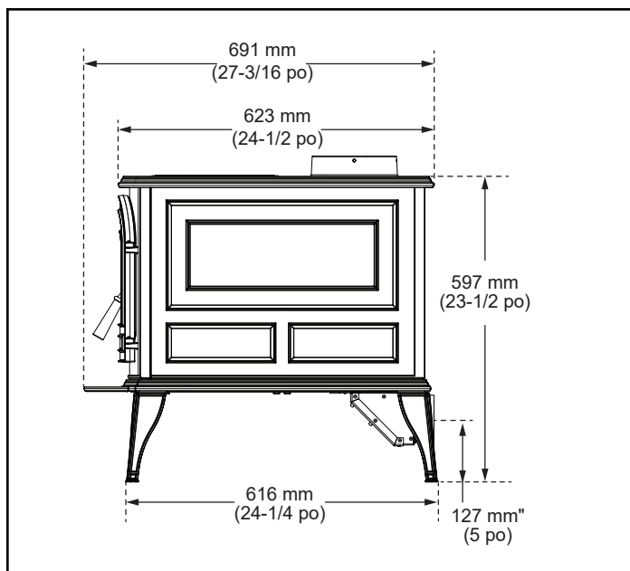
Figure 3.2 – Vue latérale
